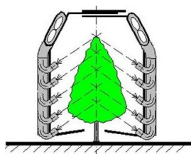
Rys. 9. Systemy emisji powietrza i cieczy w opryskiwaczach sadowniczych: A – radialna; B – pozioma; C – kierowana; D – opryskiwacz tunelowy
