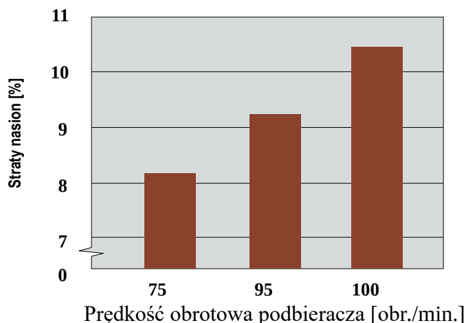
Rys. 12. Straty nasion rzepaku powodowane różnymi prędkościami obrotowymi podbieracza pokosów (Szot i wsp. 1991)
