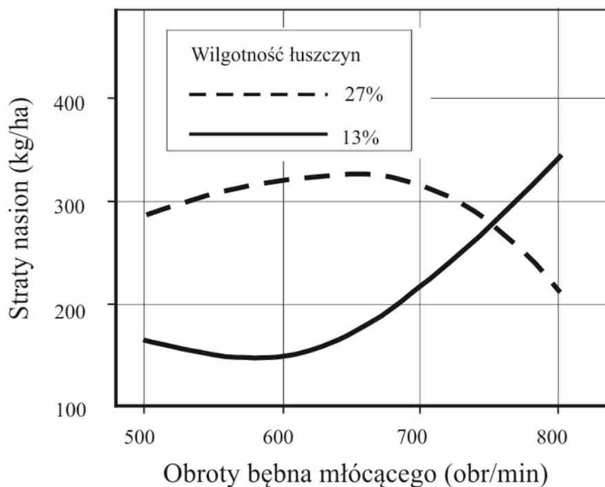
Rys. 13. Wpływ obrotów bębna młójącego i wilgotności łuszczyń na wielkość strat nasion (Szot i wsp. 1991)
