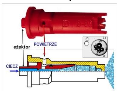
Rozpylacz płaskostrumieniowy eżektorowy
