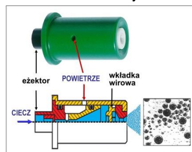
Rozpylacz wirowy eżektorowy
