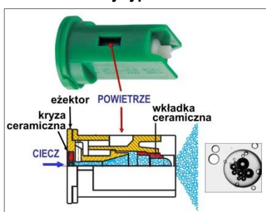
Rozpylacz płaskostrumieniowy eżektorowy typu KOMPAKT
